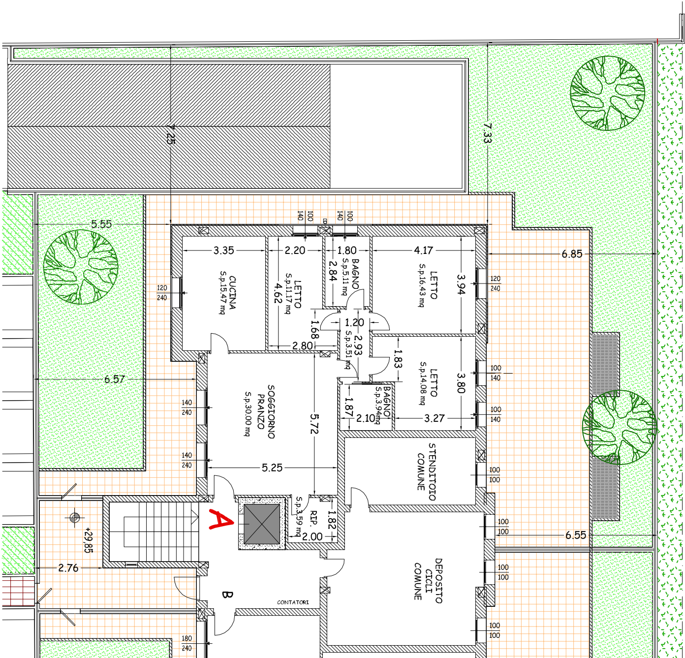
Pianta Quotata
