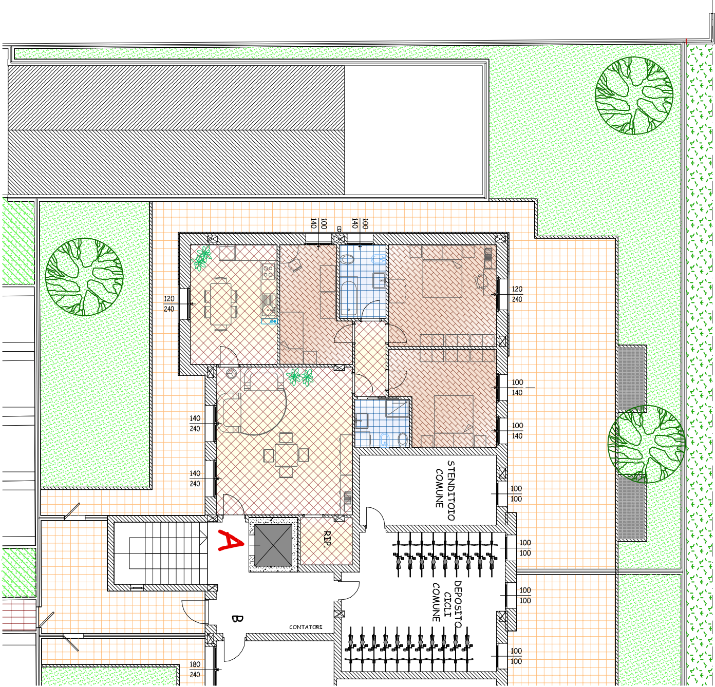
Pianta Arredata
